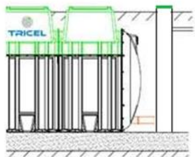
Exemple de poste de relevage en sortie de filtre compact Seta
